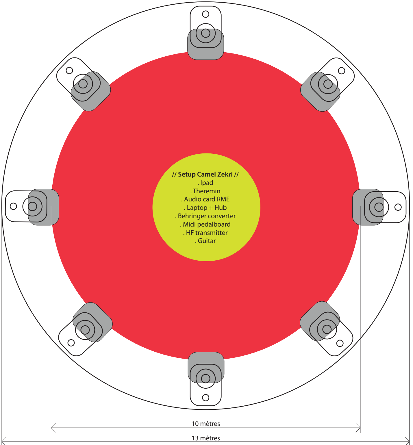
Diffusion Focal Alpha 80 Monitor (X8)
